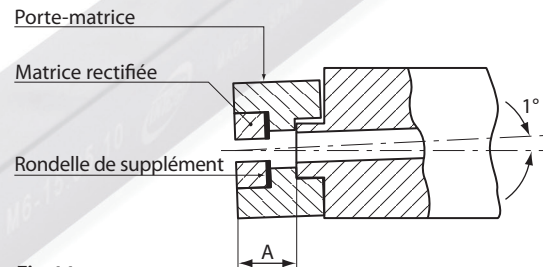
Fig.11 Porte-matrice avec matrice réaffûtée.
