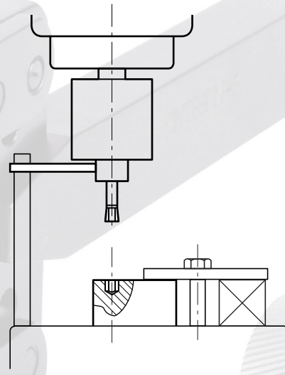
Fig.8 Application du levier auxiliaire sur fraiseuse ou perceuse.
