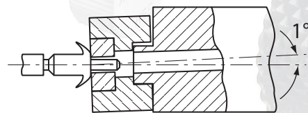
Fig.2 Exemple de coupe progressive externe.
