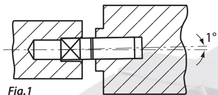
Fig.1 Exemple de coupe progressive interne.
