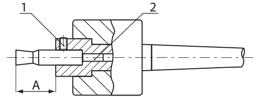
Fig.9 Réglage de la longueur de la broche.
