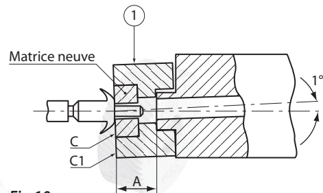
Fig.10 Porte-matrice avec nouvelle matrice.
