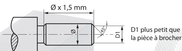
Fig.6 Exemple de brochage externe.
