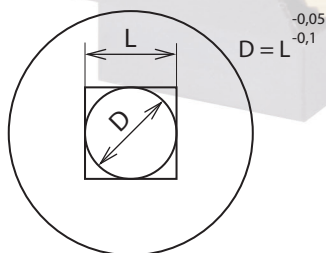
Fig.3 Exemple de pièce avec D < L
