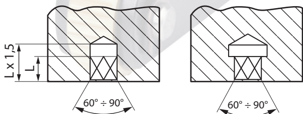
Fig.5 Profondeur d'orifice et angle d'entrée.
