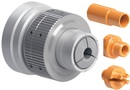
Mandrin de pince B45 automatique type FNP-KAH-B45, avec une limitation de chemin, pour des pinces tirées B45, version axe-fix.
